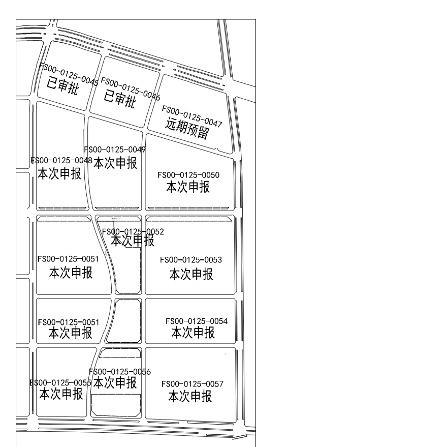
总平面图 1:1000
