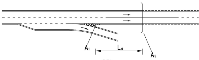
(d) 隧道入洞口与分流点距离示意图
