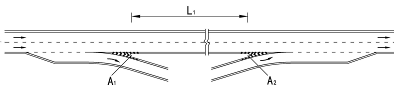
(a) 隧道内相邻“出-出”示意
