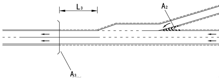
(a) 隧道出入口与合流点距离示意图
