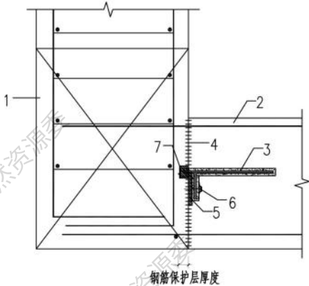
1—主体结构暗梁；2—附属（区间）结构；3—卡槽型高分子涂层止水带； 4—水泥基渗透结晶防水涂料或其他界面剂；5—固定用配套胶；6—螺栓；7—槽口 图 21 主体结构与附属（区间）结构接口接缝防水构造图
