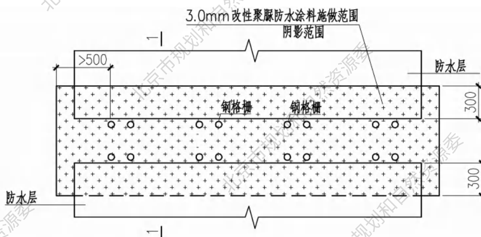
图 16 钢筋格栅穿防水层构造平面图配图
