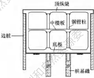
图 4 盖挖逆作法
