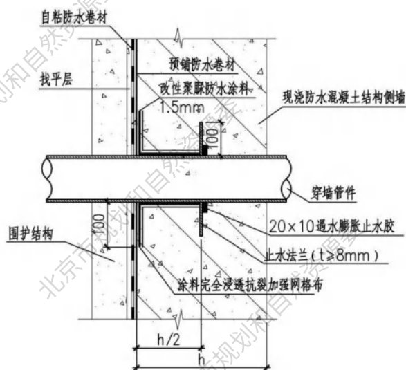
图 24 穿墙管防水构造图
