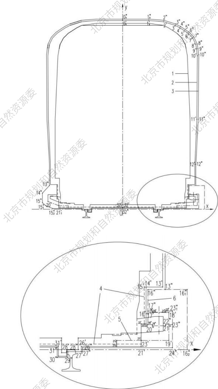
图 B.0.1-3 B 1 型 DC1500V 下部受流车区间车辆限界和区间直线地段设备限界
