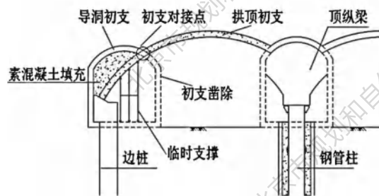
图7 拱部作法示意图
