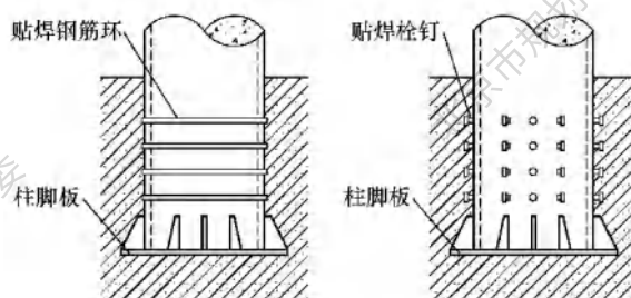
图2 插入式柱脚
