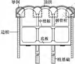
图 5 洞桩逆作法
