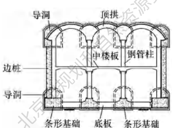
图 6 洞桩逆作法
