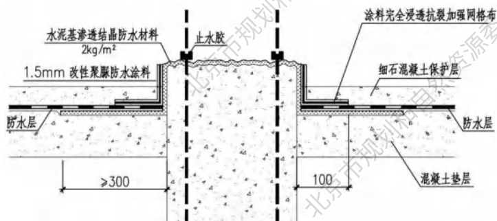
图 23 桩头防水构造图
