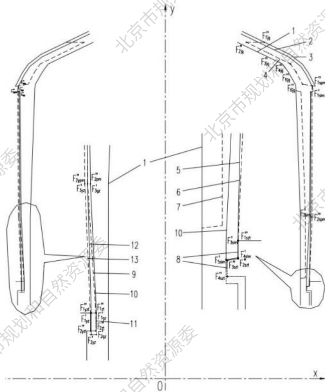
图 A.0.2 A 2 型车计算站台长度范围内附加车辆限界、直线站台及站台屏蔽门限界、检修库高低平台限界 1—计算车辆轮廓线；2—区间车辆限界；3—直线设备限界；4—检修库高平台限界；5—塞拉门车停靠开门附加车辆限界；6—塞拉门车站台屏蔽门限界；7—塞拉门车开门计算车辆轮廓线；8—塞拉门车站台和检修库低平台限界；9—非塞拉门车站台屏蔽门限界；10—停站进出站附加车辆限界；11—非塞拉门车站台和检修库低平台限界；12—越行附加车辆限界；13—越行站台及站台屏蔽门限界
