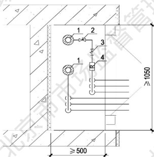
图 12.0.4-2 公共管井尺寸示意图二
