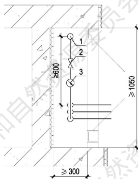
图 12.0.6-1 单排水表安装尺寸示意图
