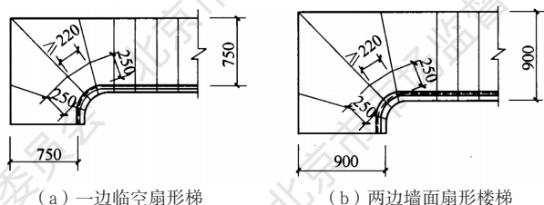
图 1 一边临空与两侧有墙的楼梯净宽要求不同
