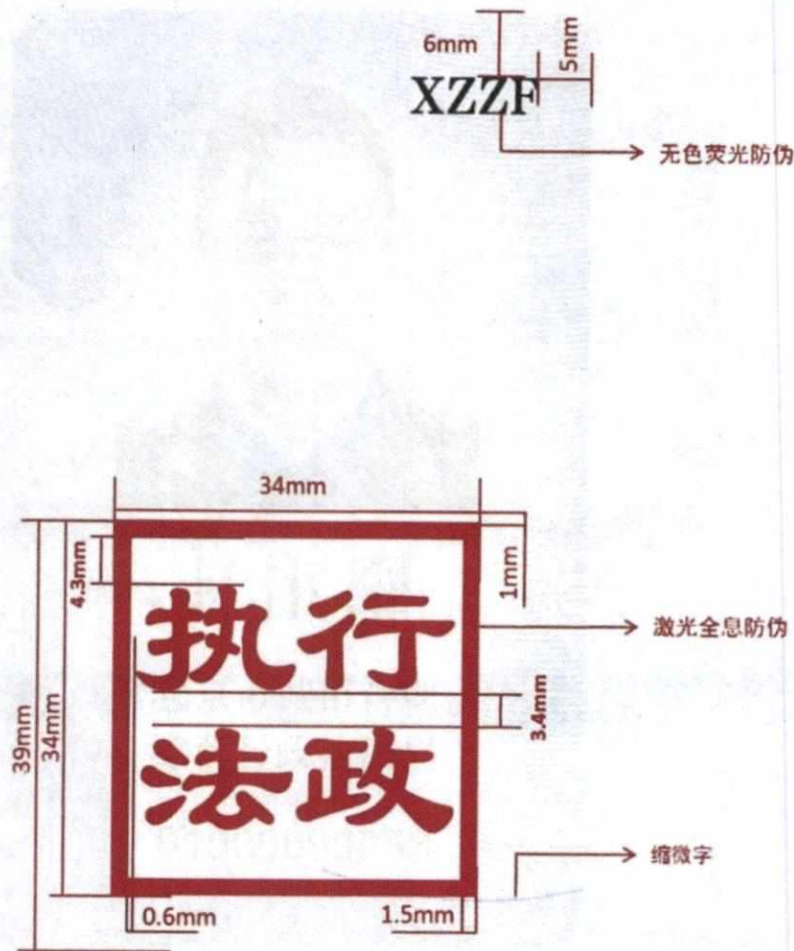
图 5：防伪标识各要素坐标及尺寸
