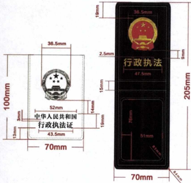
图3：皮夹各要素坐标及尺寸
